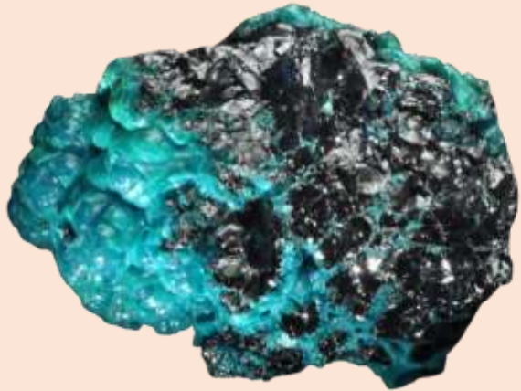
HETEROGENITA Hidròxid de cobalt
