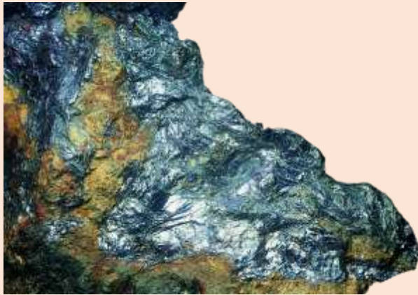
MOLIBDENITA Sulfur de molibdè
