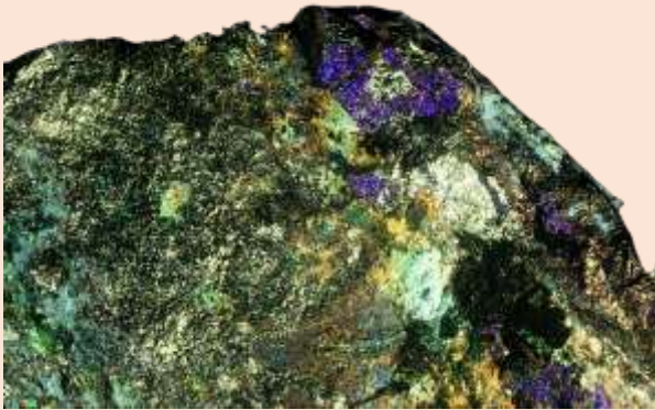
CALCOPIRITA Sulfur de coure amb seleni
