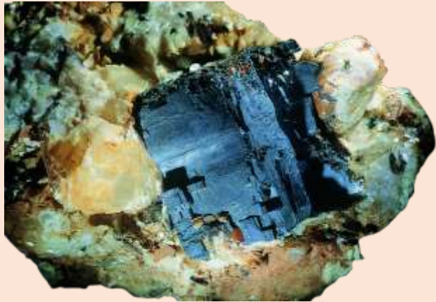
GALENA Sulfur de plom
