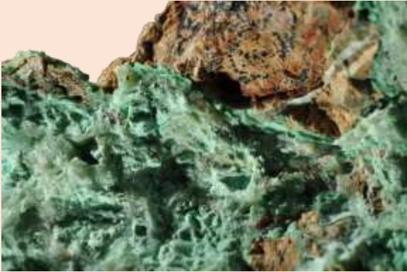
NEPOUÏTA Silicat de níquel
