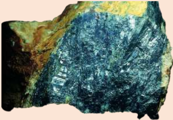
ESTIBNITA Sulfur d'antimoni
