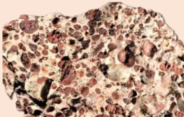
BAUXITA Hidròxids d'alumini
