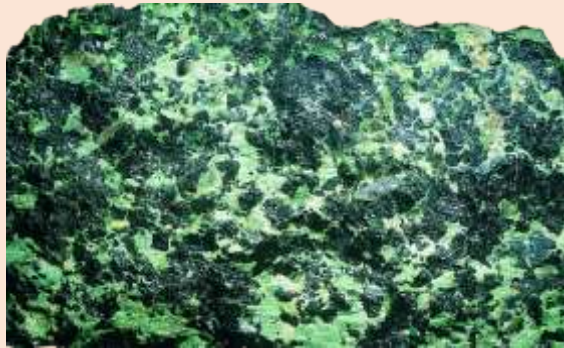
CROMITA Òxid de crom
