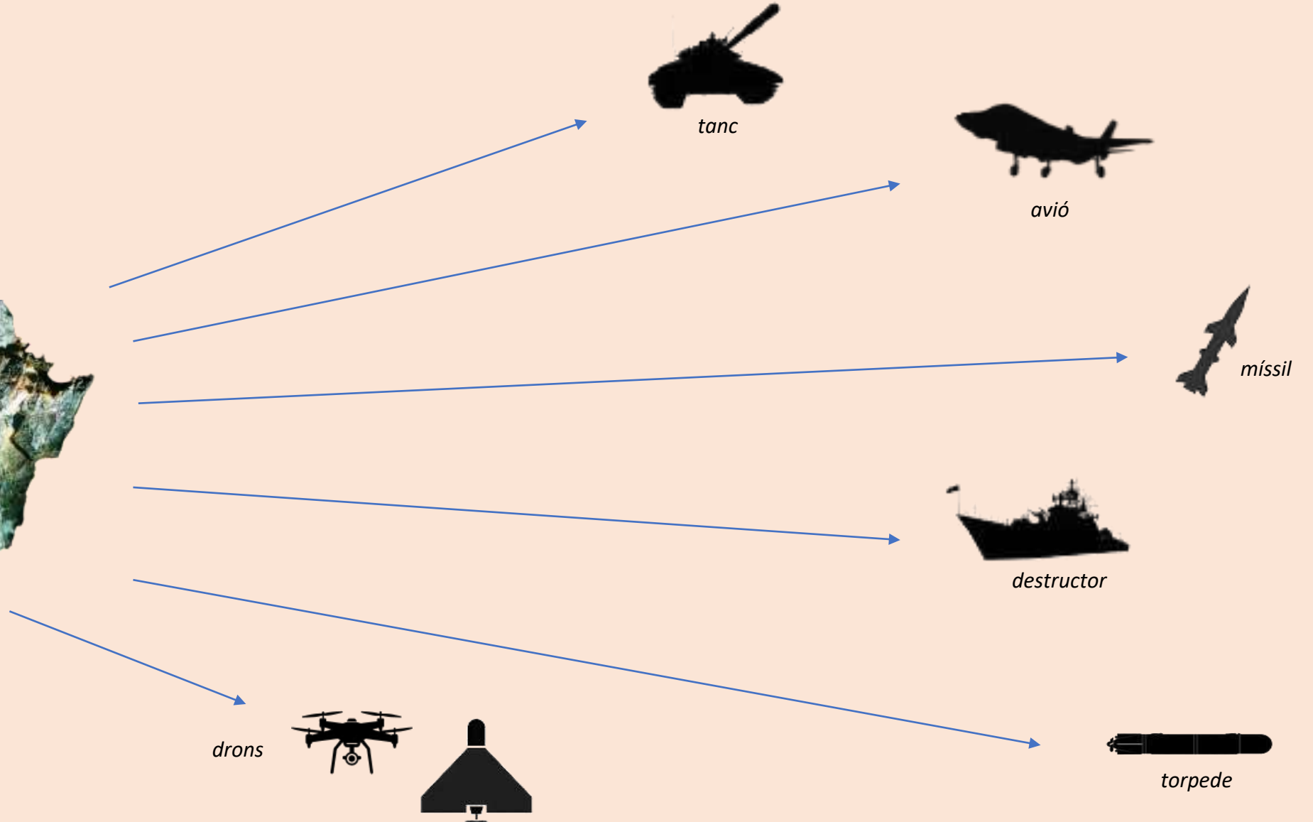
CASSITERITA Òxid d'estany
