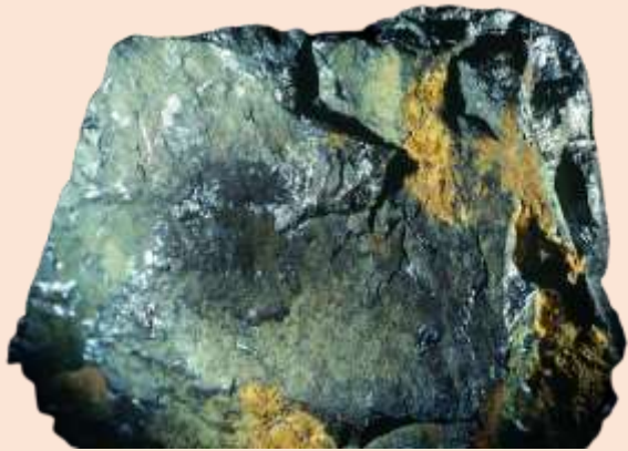
ILMENITA Òxid de titani i ferro
